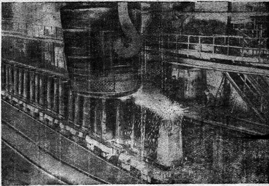
Внутризаводской транспорт, обслуживая цехи комбината, осуществляет все виды перевозок. На снимке: железнодорожный состав изложниц принимает плавку.
