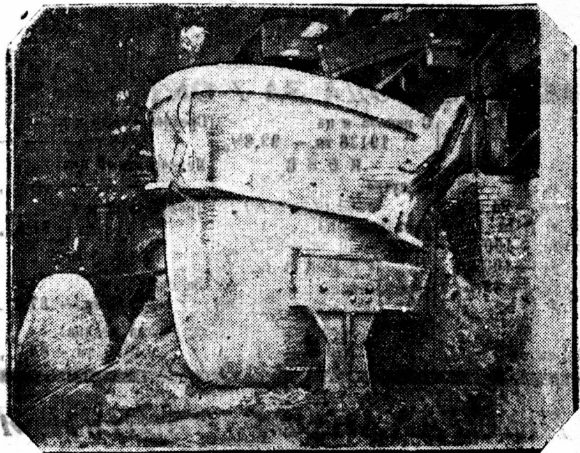
На печи № 11 постаменты залиты шлаком. Чаша стоит не на постаменте, а на шлаке. Фото Новикова.
