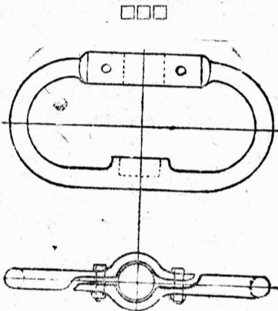
Схема ручки, сделанной тов. Гальяновым.
