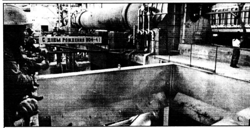
Вращающаяся печь № 4...
