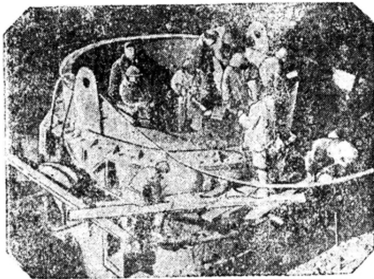
Сборка разливочного козла на мартене
