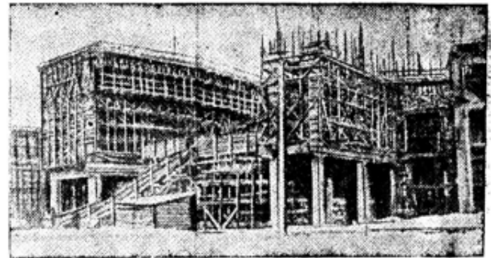
НА СНИМКЕ: Общий вид строительства Безымянской теплоэлектростанции. Фото Н. Славина. Фото-Клише ТАСС.
