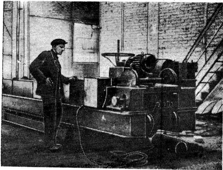
Слесарь третьего мартеновского цеха Иван Васильевич Щедрин является активным рационализатором. На протяжении последних лет он внес много предложений. Последнее из них, наиболее важное, — машина для скачивания шлака из миксера. Рационализатор сам и смонтировал эту машину. Она будет установлена у миксера при оборудовании площадки. На снимке: И. В. Щедрин у изготовленной им машины для скачивания шлака.
