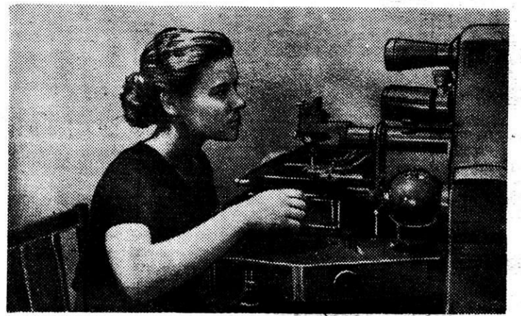
Спектральщица лаборатории доменного цеха Ольга Пономарева освоила новый метод анализа чугуна на спектрографе. Все анализы она делает быстро и безошибочно. На снимке: Ольга Пономарева за работой.
