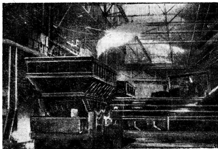
В мартеновском цехе. Загрузка сталеплавильной печи. Фото Е. Карпова.
