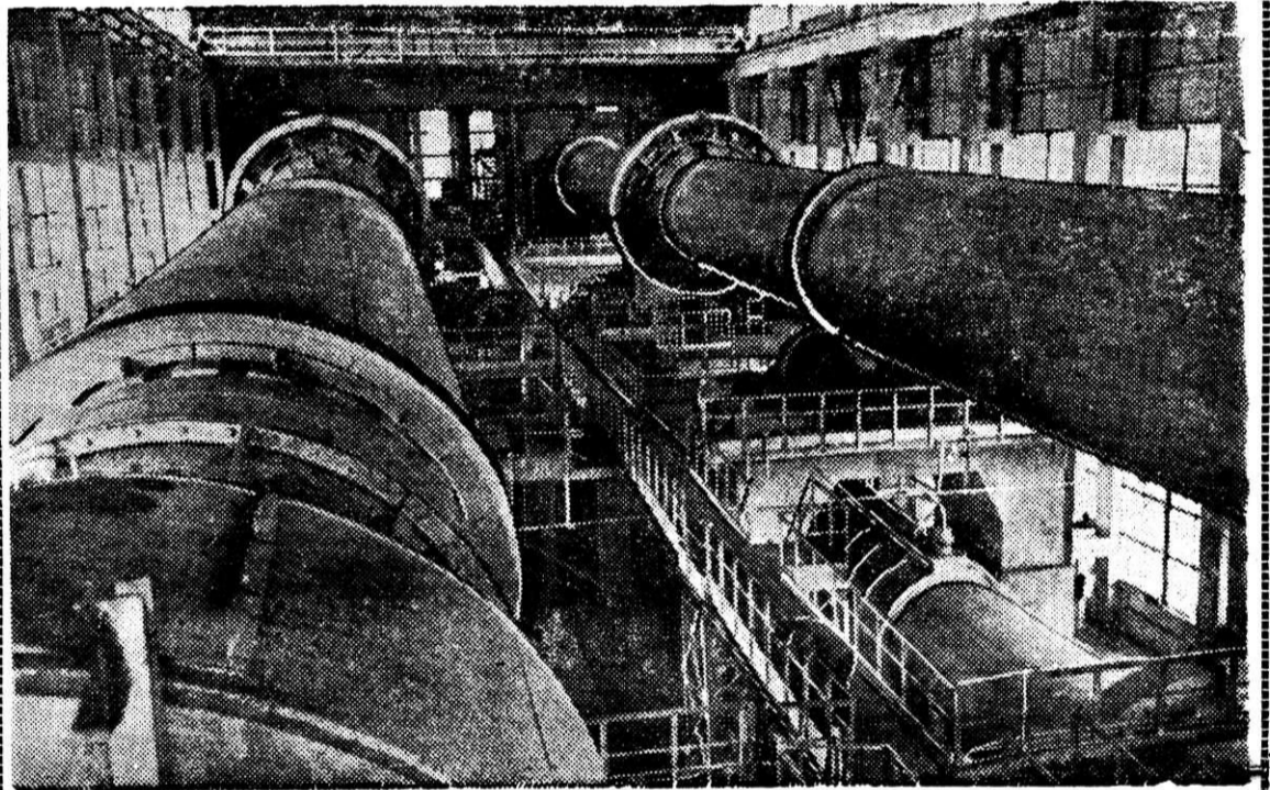
Таким будет новый огнеупорный цех.
