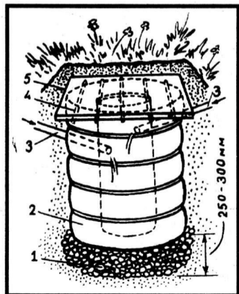
1 — крупнозернистый гравий; 2 — автомобильная покрышка; 3, 4 — сливные трубы; 5 — крышка.
