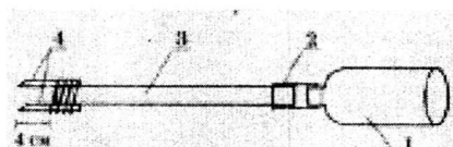
Подкормщик: 1 — бутылка, 2 — шланг, 3 — труба, 4 — «зубья-рыхлители».
