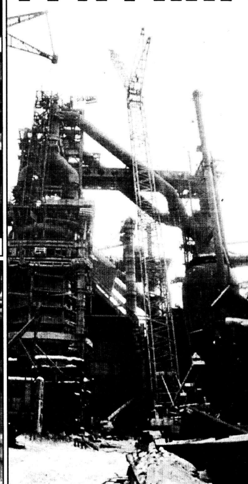
Доменная печь № 2.
