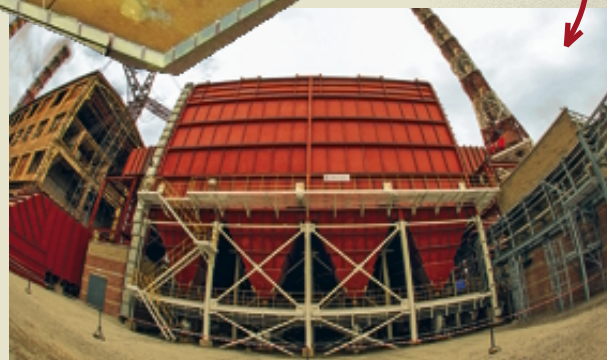
Комплекс по очистке агломерационного газа сероулавливающей установкой
