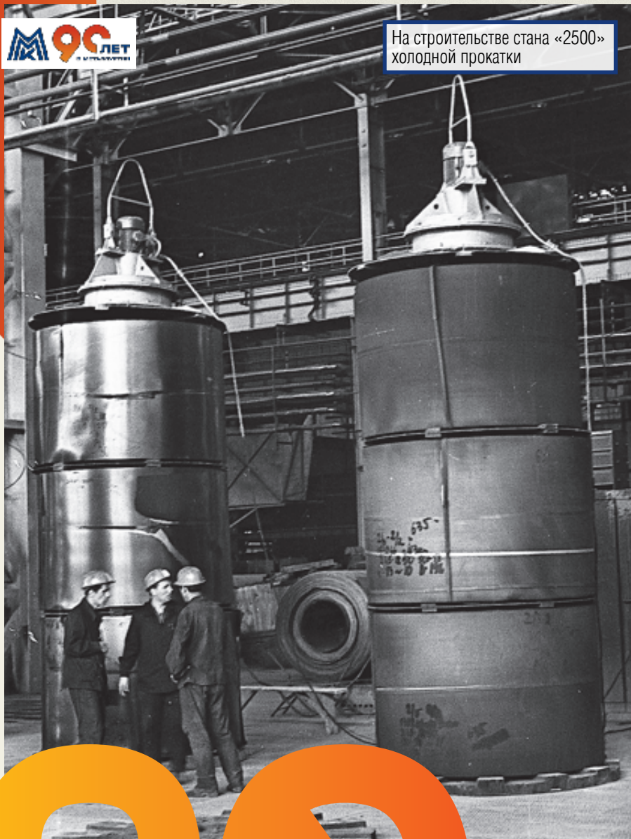
Монтаж электрооборудования на стане «2500» холодной прокатки
